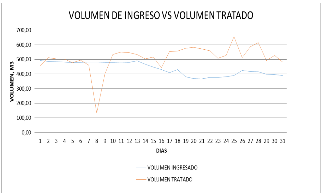
Diagrama 2: Volumen de ingreso vs volumen tratado
